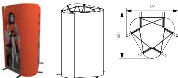
2225 h x 1660 w x 1500 d mm
